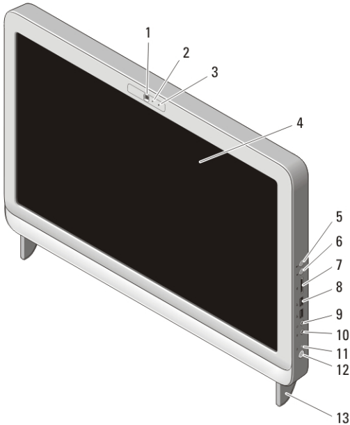
図 1. 正面図
